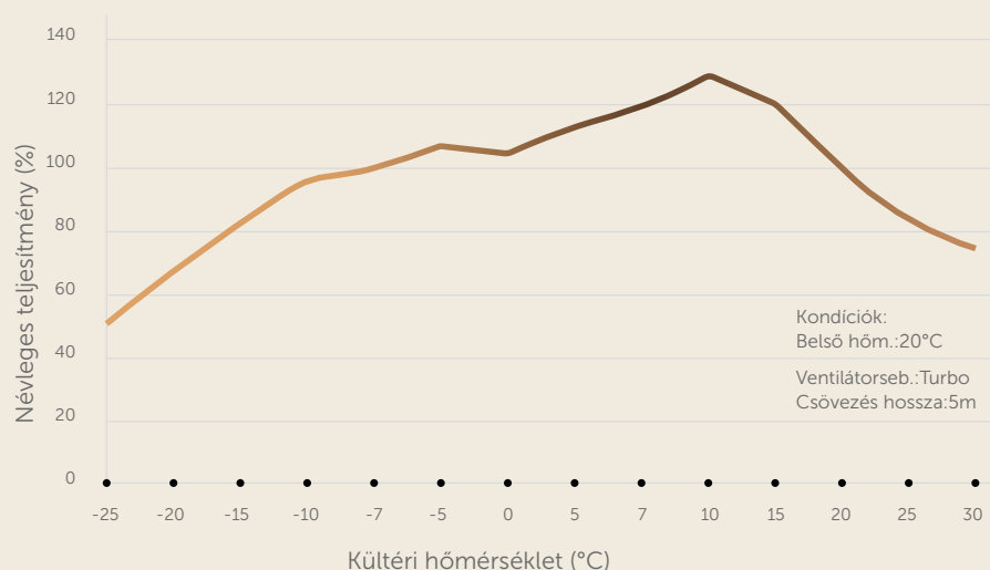
2,7 és 3,5 kW-os Comfort Pro fűtési teljesítménye különböző külső hőmérsékletek mellett
